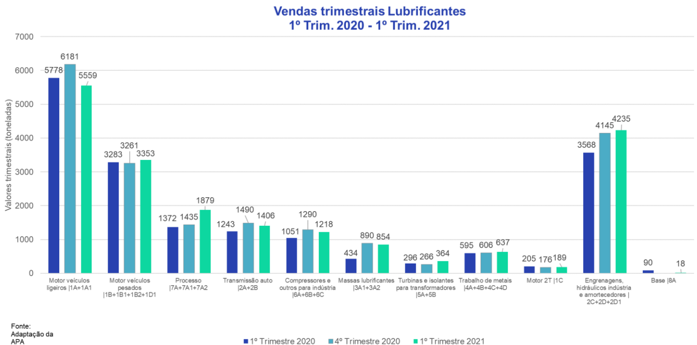
Figura 1 - Consumo de Lubrificantes.
